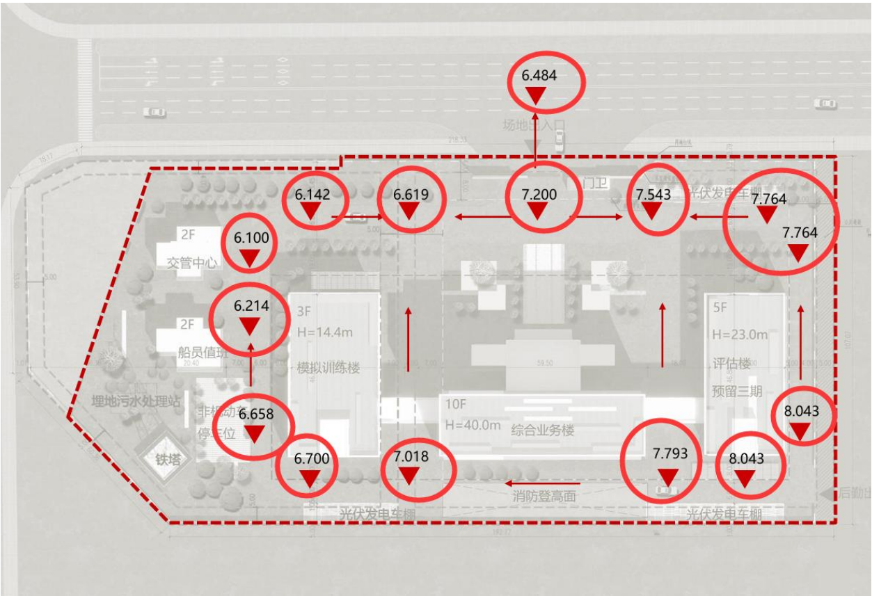
调整前总图竖向标高
