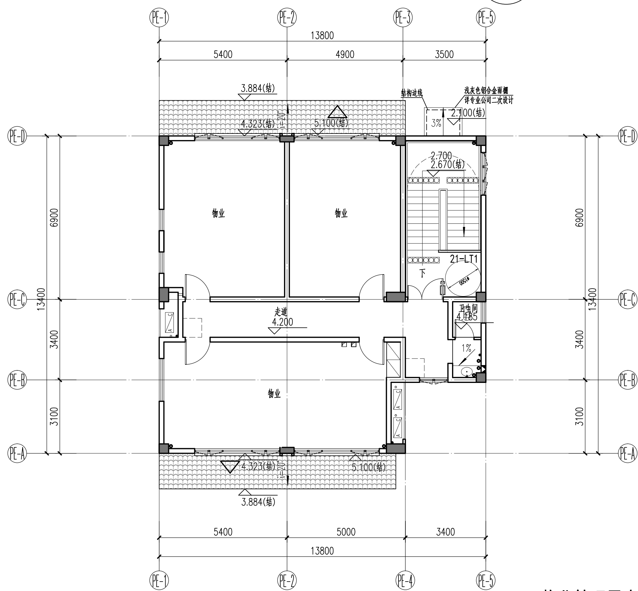
21#物业管理用房二层平面图 1:100 二层建筑面积: 174.72m 2
