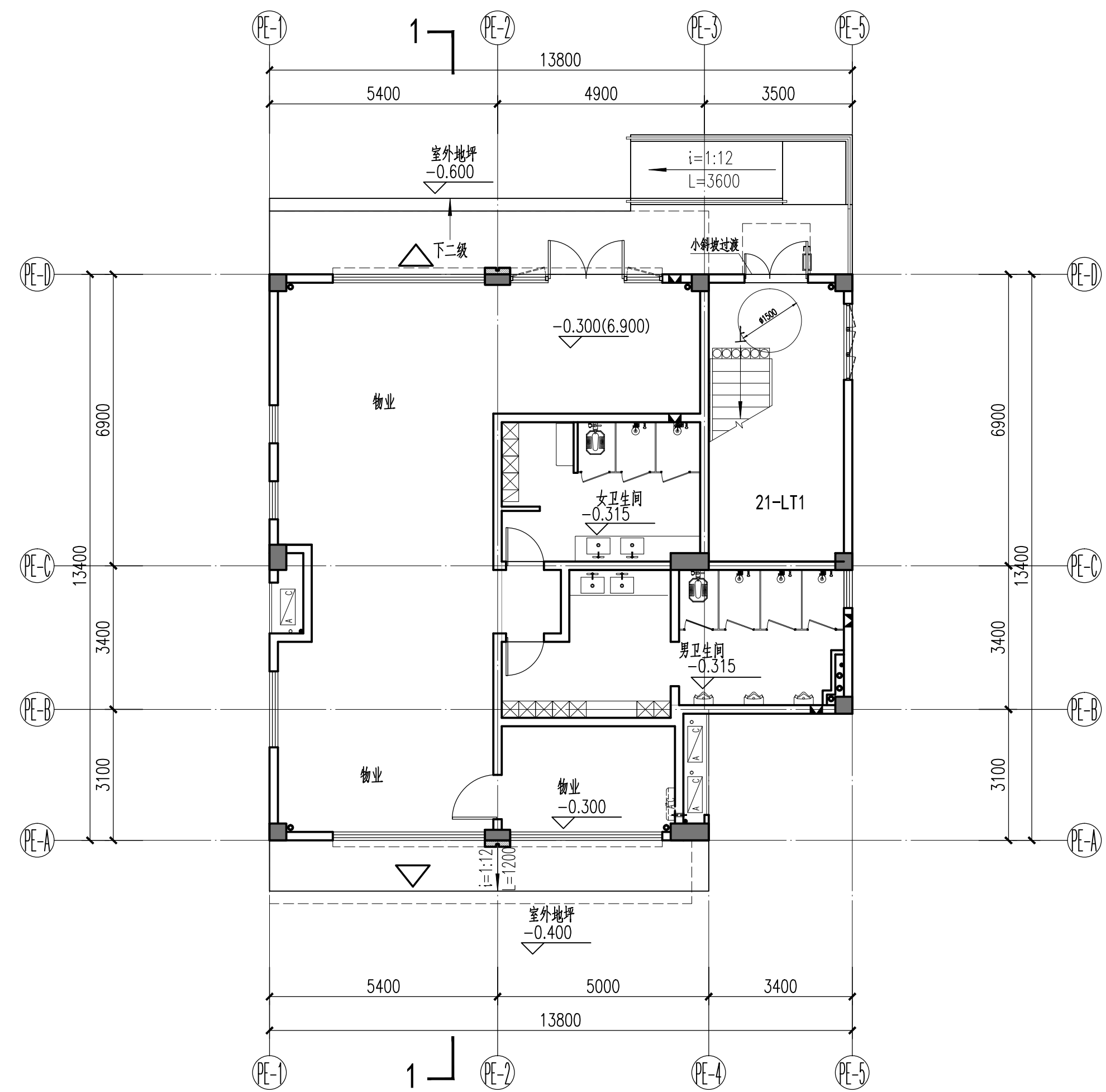
21#物业管理用房首层平面图 1:100
