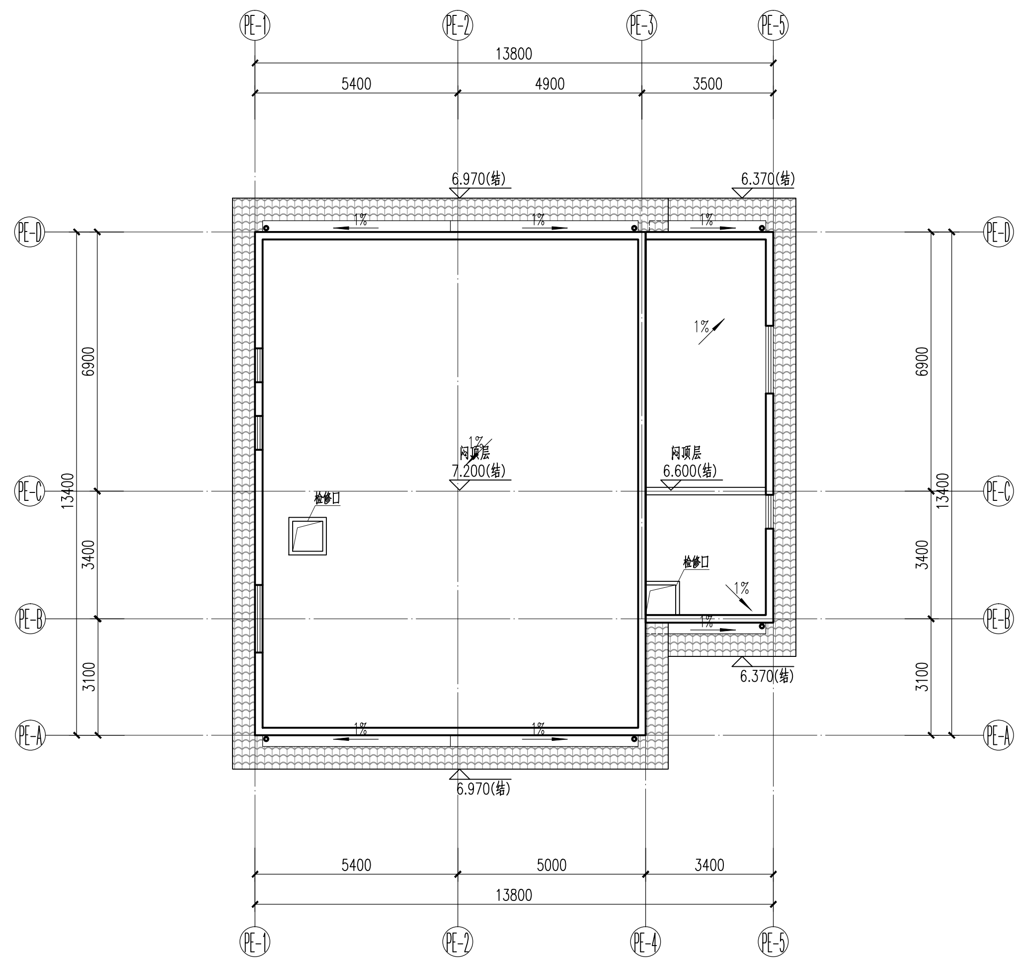
21#物业管理用房闷顶层平面图 1:100
