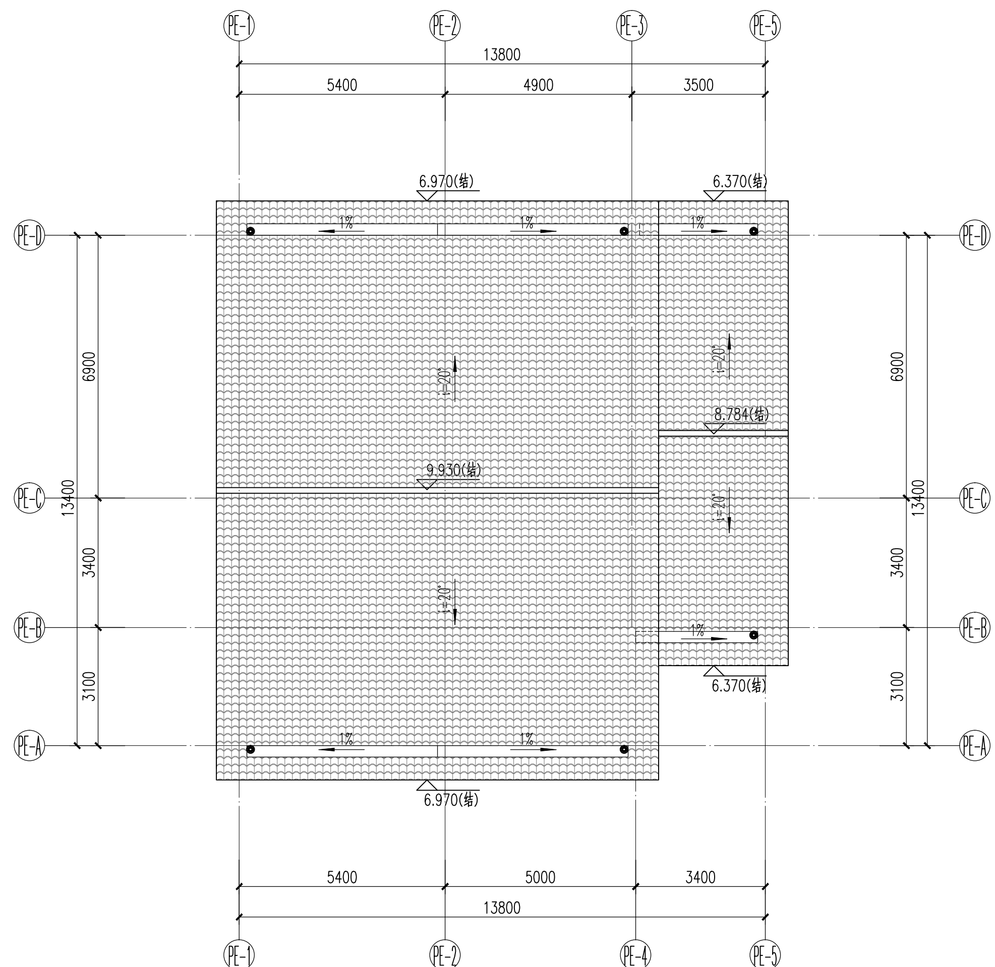
21#物业管理用房屋面层平面图 1:100
